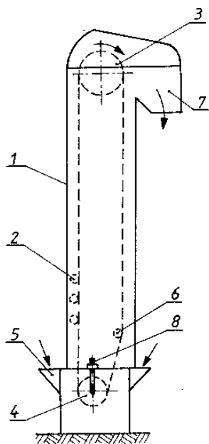
Rys. 2.6. Przenośnik kulekowy
