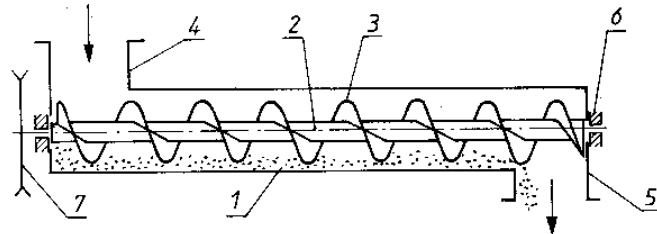
Rys. 2.10. Przenośnik ślimakowy 1 — koryto, 2 — wał, 3 — taśma, 4 — kosz zasypowy, 5 — wylot, 6 — łożysko, 7 — koło pasowe
